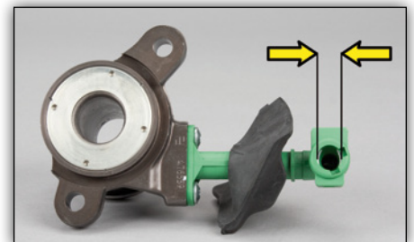
Bild 4: LuK CSC 510 0137 10 Hydraulikanschluss 12,2 mm
