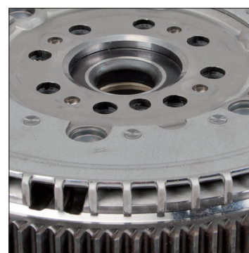
Bild 2: Geberring neue Ausführung
